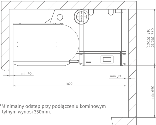
Widok z góry, minimalne odstępy: (podłączenie komina z góry*)
