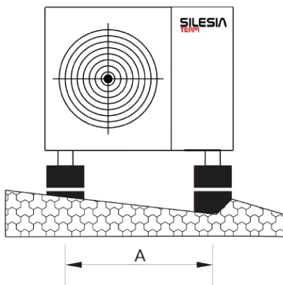
A – pompy 10 – 13 kW rozstaw 1100mm A – pompy 16 – 25 kW rozstaw 1220mm
