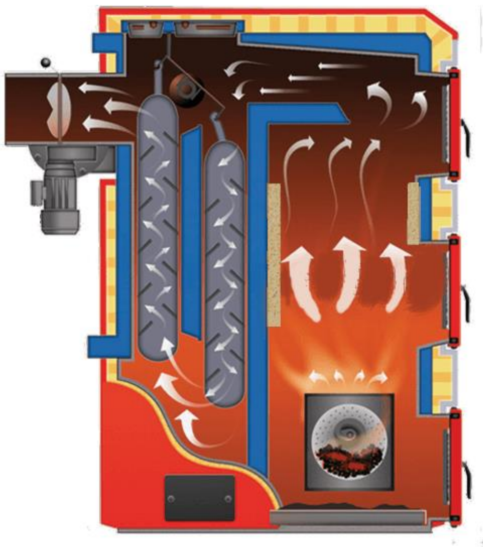
Rysunek 7. Schemat blokowy kotła typu Bio Bio Pellmax
