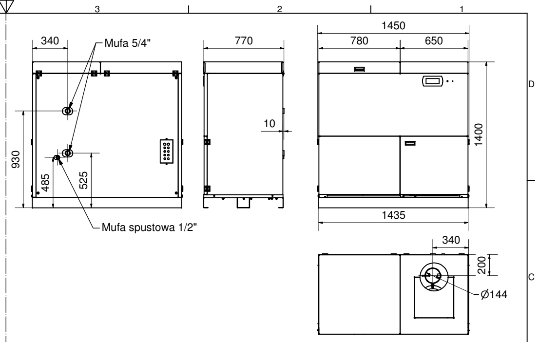
EG Pellet 10-25 kW powiększony - lewy
