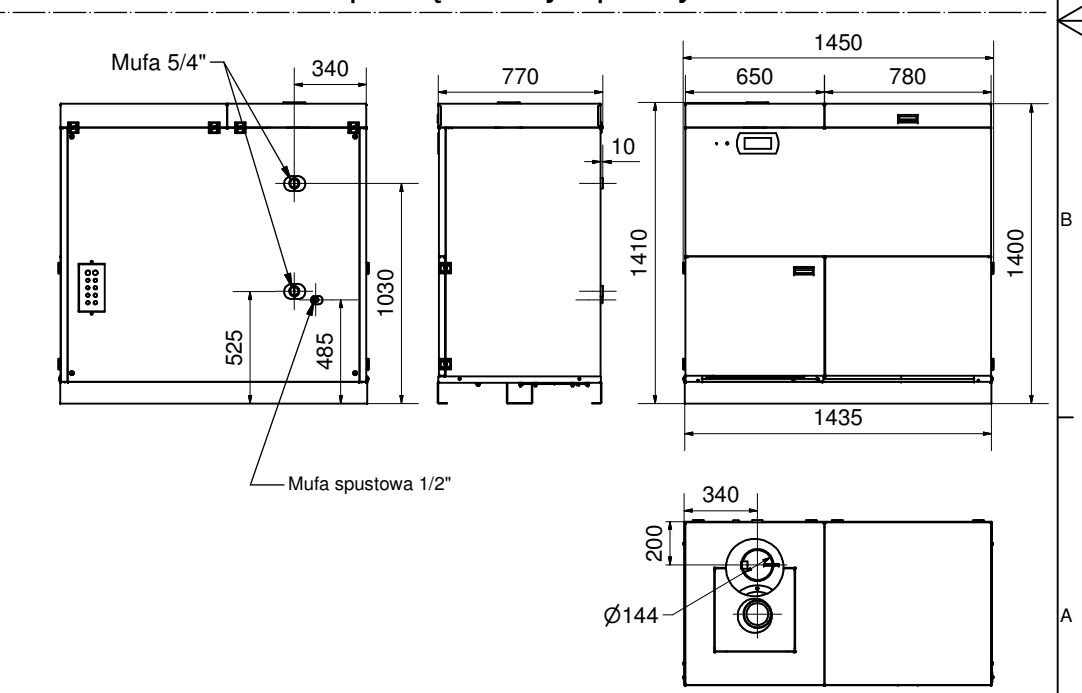
EG Pellet 40 kW powiększony - prawy
