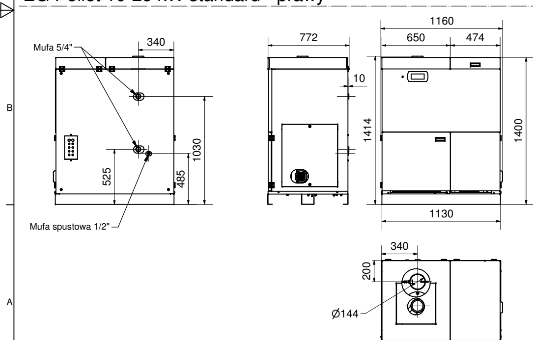
EG Pellet 40 kW standard - prawy
