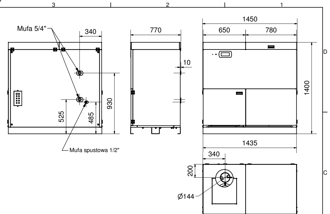
EG Pellet 10-25 kW powiększony - prawy
