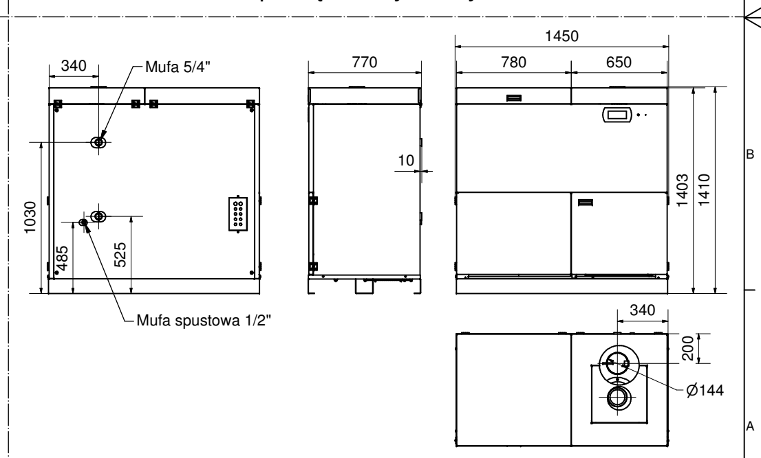
EG Pellet 10-25 kW powiększony - lewy
