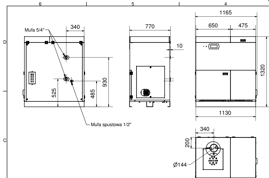
EG Pellet 10-25 kW standard - prawy
