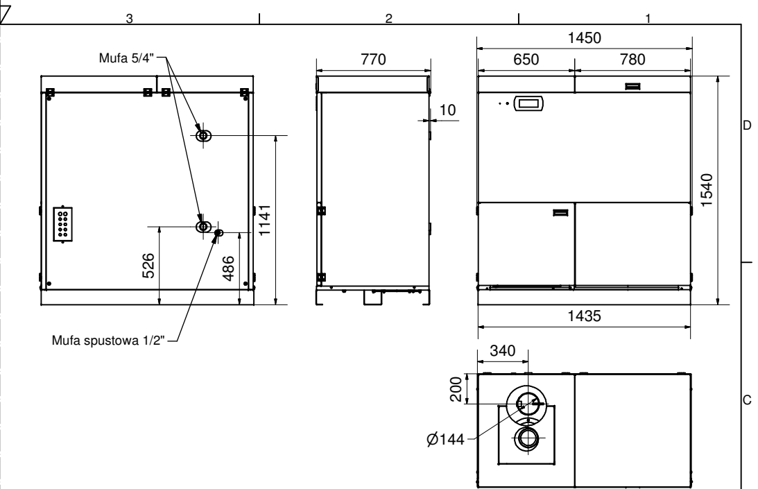
EG Pellet 60 kW powiększony - prawy
