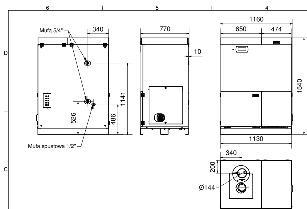
EG Pellet 60 kW standard - prawy
