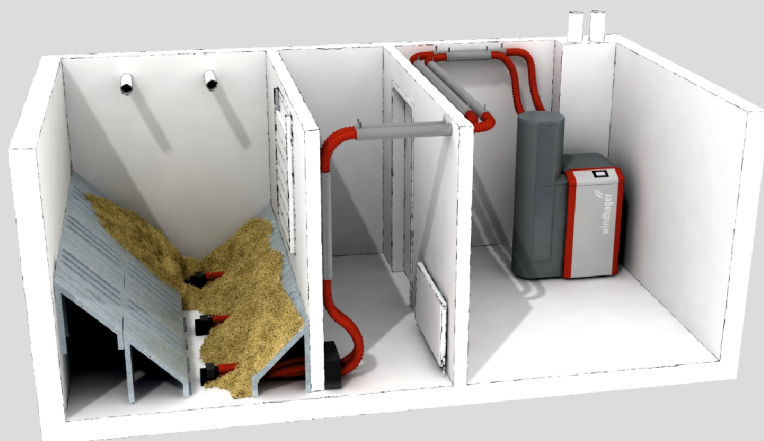
Kocioł BioWIN 2 TOUCH z 3-ma sondami ssącymi i jednostką zmieniającą
