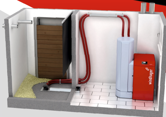
Kocioł BioWIN 2 TOUCH z 1-sondą ssącą i przegarniaczem
