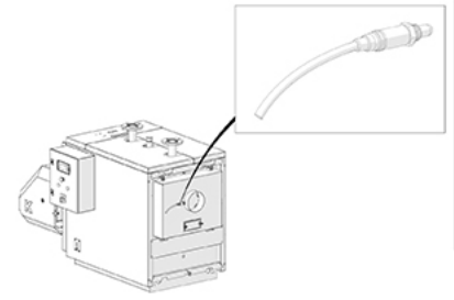
sonda lambda
