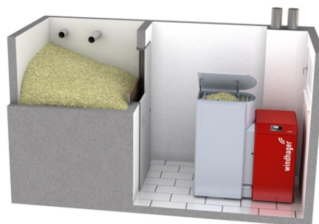
Kocioł BioWin2 z 1-sondą ssącą i przegarniaczem
