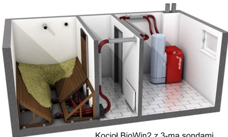
Kocioł BioWin2 z 3-ma sondami ssącymi i jednostką zmieniającą
